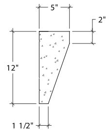
JAMB SECTION
