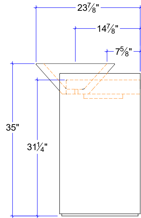
RIGHT ELEVATION
