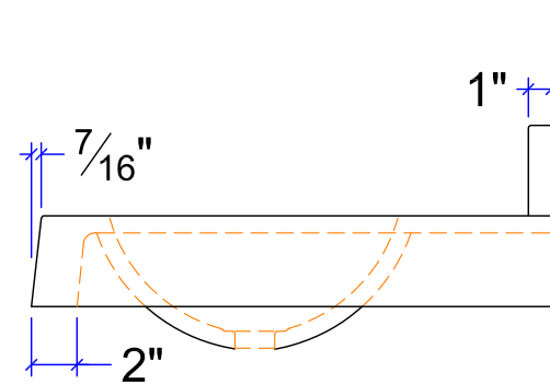
RIGHT ELEVATION
