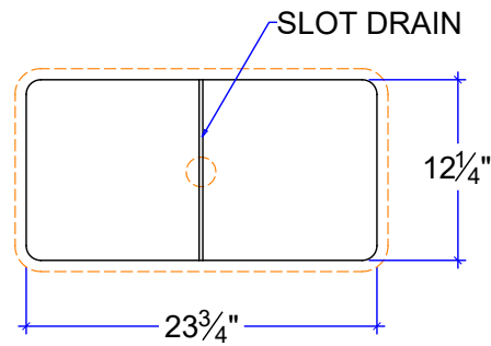
CS-2312-SD 7 1/2" DEEP
