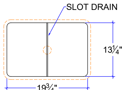
CS-1913-SD 7" DEEP
