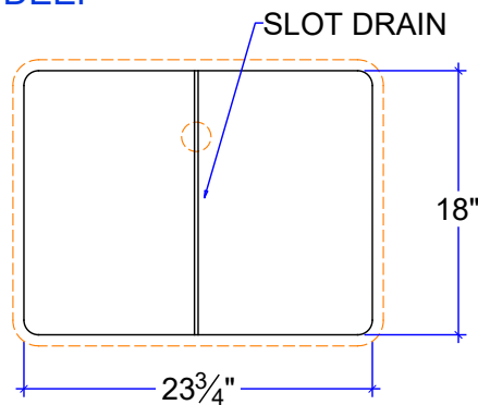
CS-2418-SD 7 1/2" DEEP
