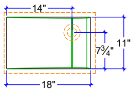
CS-1811 * 18" x 11" x 5"
