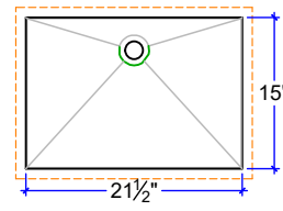
CS-2215 ^ 21 1/2" x 15" x 3 1/4"
