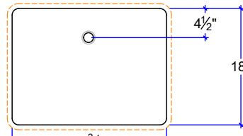
CS-2418 23 3/4" x 18" x 7 1/2"
