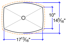
CS-1714* ^ 17 13/16" x 14 5/16" x 4 1/2"
