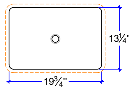
CS-1913* 19 3/4" x 13" x 7"
