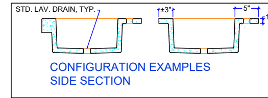
"CRESCENT" SINK + CS-1813, CS-1913, CS-2117 SIDE SEC.
