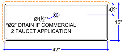
CS-4215-FB ^A.D.A. COMPLIANT 42" x 15" x 5 1/4"
