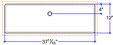
CS-3812-FB ^ 37 1/16" x 12" x 5"
