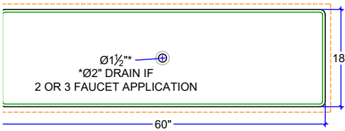
CS-6018-FB 60" x 18" x 6"
