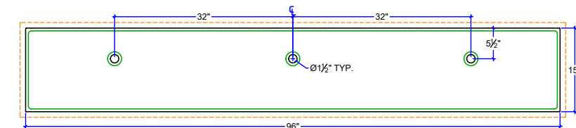
CS-9615-FB ^A.D.A. COMPLIANT 96" x 15" x 4"
