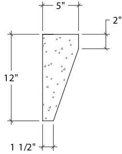
JAMB SECTION
